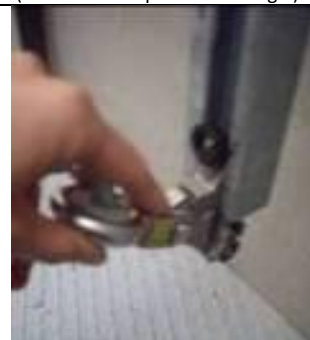
Figuras 21 – Extracción del carril del dispositivo anticaídas deslizante
