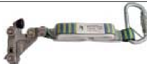
Figura 4.- Dispositivo anticaídas antideslizante Tipo AL-D (con dissipador de energía)
